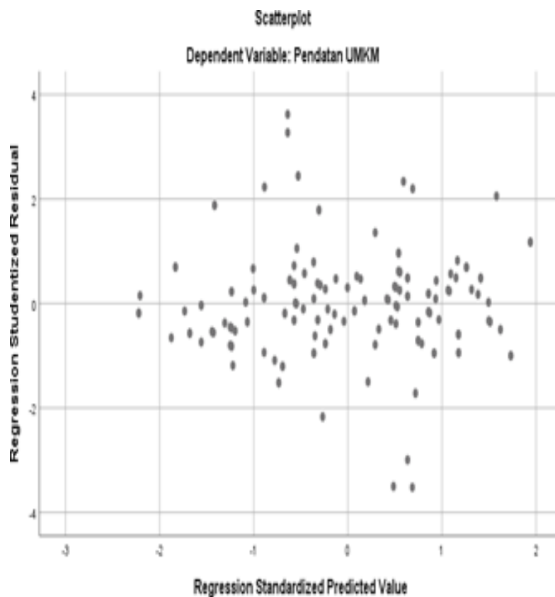
Gambar 2 Scatterplot Uji Heteroskedastisitas
