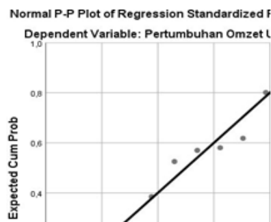
Gambar 3. Output P-Plot, 2026
