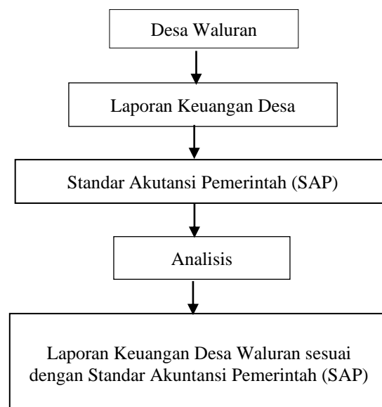
Gambar 1. Kerangka Pemikiran
